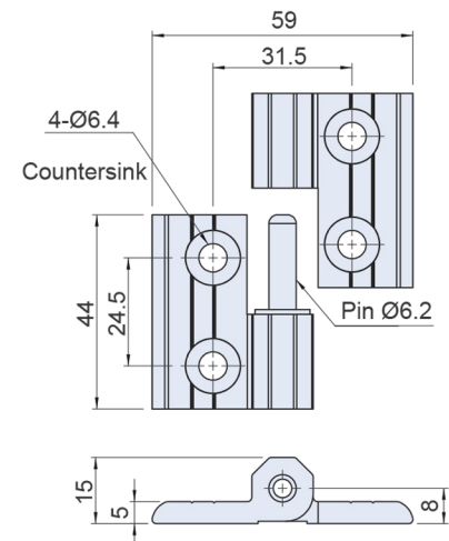
Right Opening Unit:mm
