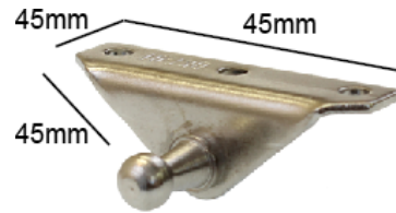
gskbrkt01
